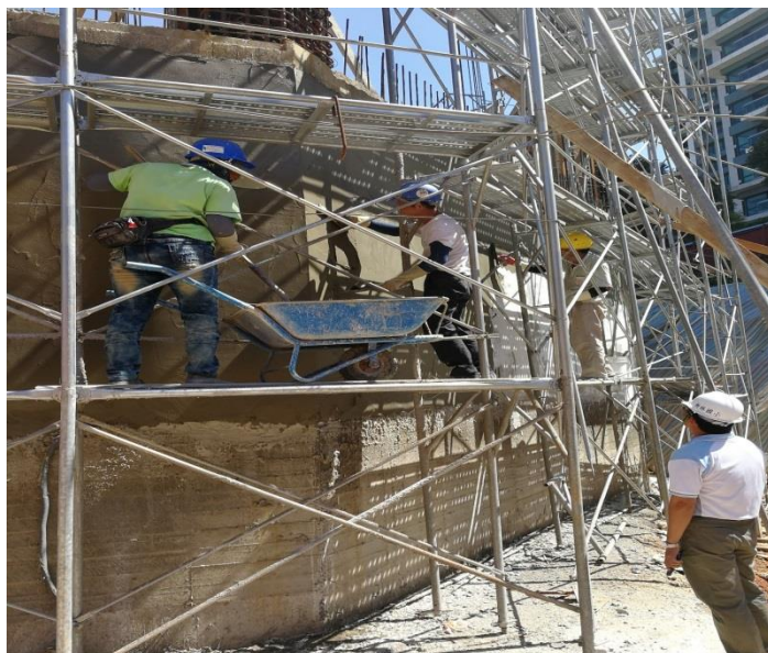
照片說明：AB 棟 B1 外牆防水工程
