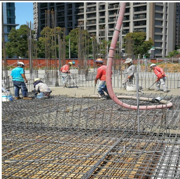
照片說明：AB 棟一樓基礎版澆灌
