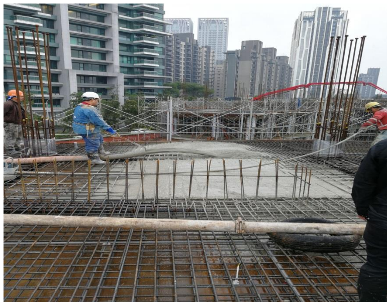
照片說明： AB 棟 3 樓版澆置
